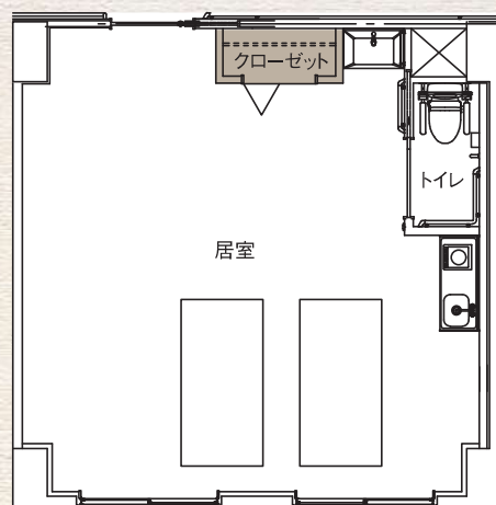
34.54㎡居室
